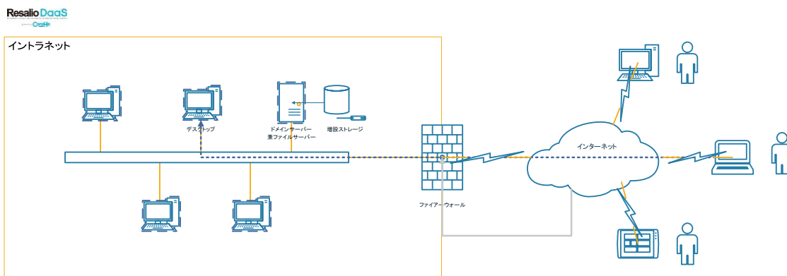
Resalio DaaS の構成図
